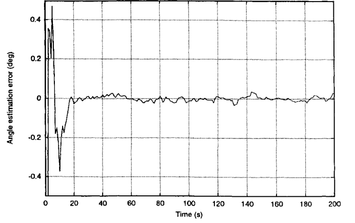
d) Roll angle estimation error
